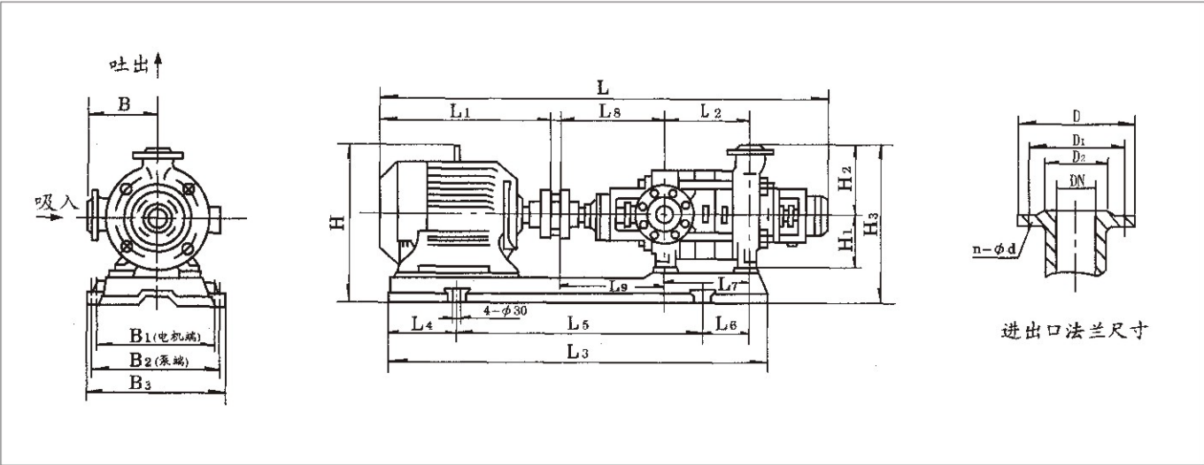
外形及安装图
