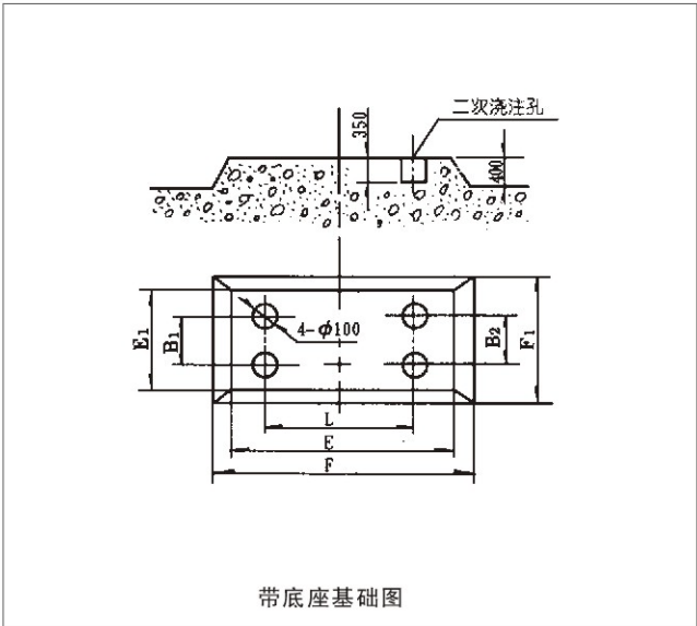
TSWA型泵基础图及联接尺寸表
